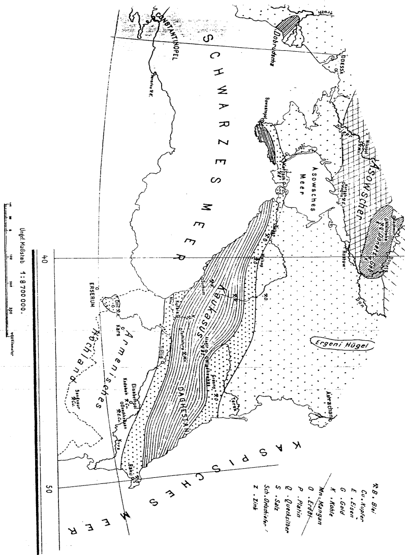
Geologische Strukturkarte von Osteuropa. Zusammengestellt von Dr. S. v. Bubnoff
