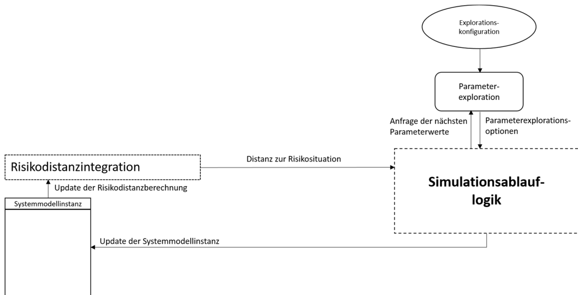
Abbildung 3-24 Übersicht über die Nutzung der Risikodistanzfunktionalität in einer Co-Simulation. Diese wird zur Exploration der Simulation in die Richtung der zu untersuchenden risikoreichen Situationen verwendet.
