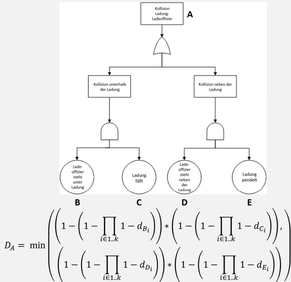
Abbildung 3-13 Struktur der Risikodistanzfunktion für den generierten Fehlerbaum zum Beispielszenario.
