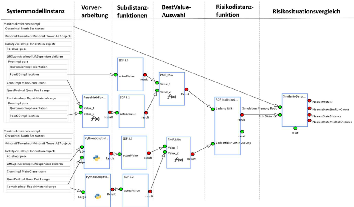
Abbildung 4-16 Ausschnitt eines Simulationsplans. In diesem wird gezeigt wie die Berechnung der Distanz zur Kollision zwischen Ladung und Ladeoffizier an Bord eines Jack-Up-Vessel konfiguriert wurde.
