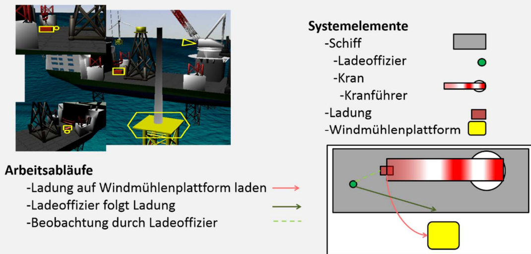
Abbildung 3-6 Übersicht über das zu analysierende Beispielszenario inklusive der zugehörigen schematischen Verhaltens- und Systembeschreibung.
