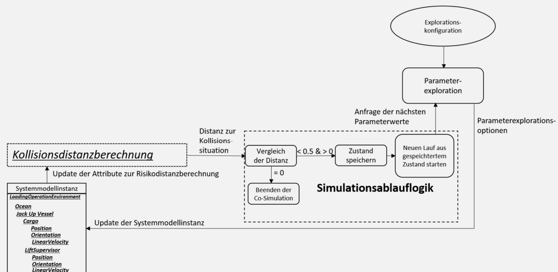
Abbildung 3-25 Übersicht über eine beispielhafte Co-Simulations-Integration, um zu einer risikoreichen Situation zu explorieren.
