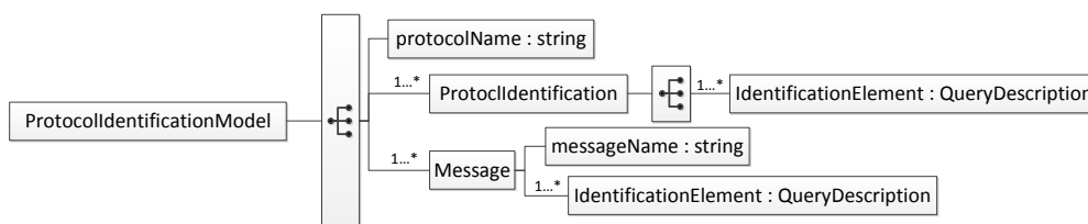
Abbildung 4.3: Schematische Darstellung des PIM
