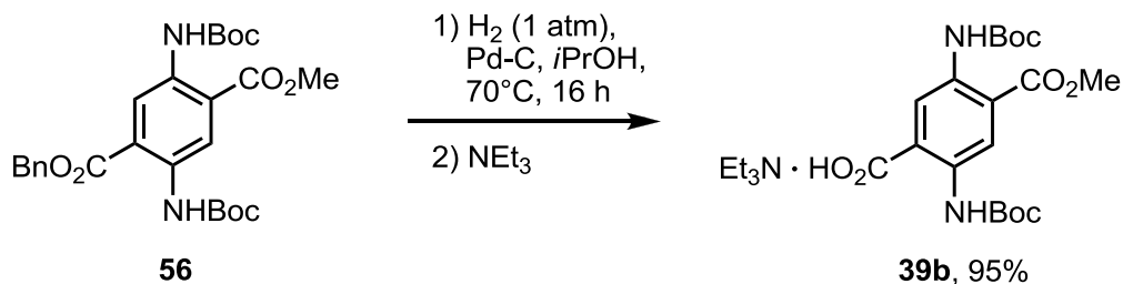
Abbildung 36: Abspaltung des Benzylesters.
