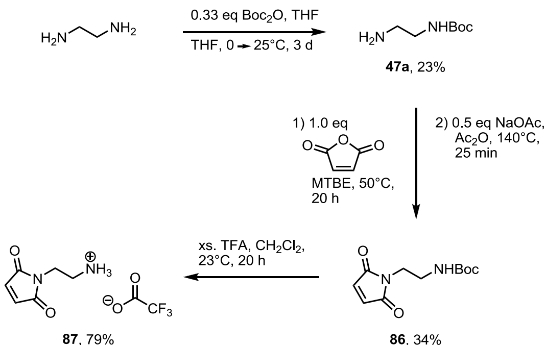
Abbildung 68: Synthese der Linkerverbindung 87 .
