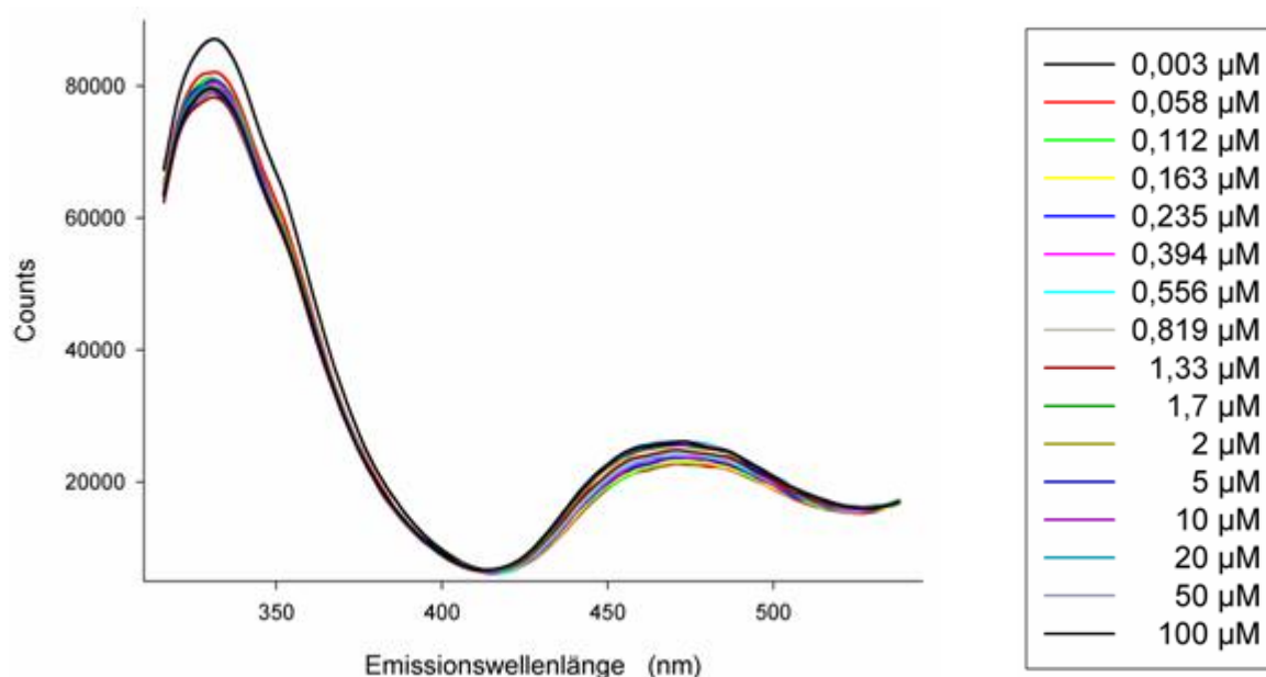
Abbildung 89: Fluoreszenzspektrum des NiWa Orange 94 am nicht-myristolierten Recoverin bei verschiedenen \text{Ca}^{2+} -Konzentrationen, \lambda_{\text{irr}} = 280 \text{ nm} .
