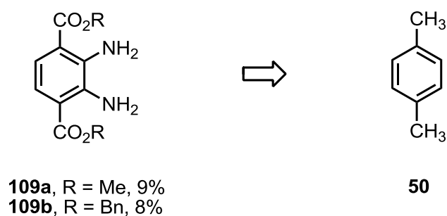
Schema VI: Retrosynthese der 2,3-Diaminodimethylester 109a und 109b
