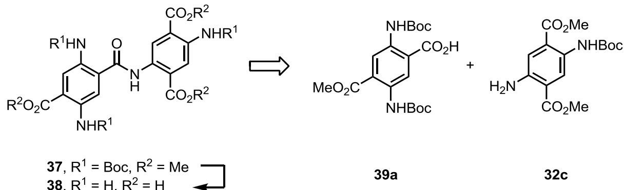
Abbildung 21: Synthese des Oligomers 38 .
