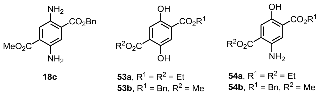
Abbildung 29: Produkt 18c und mögliche Nebenprodukte bei der Ammonolyse.
