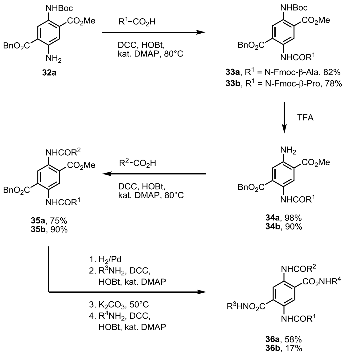
Abbildung 19: Synthese der Tetraamide 36a–b .
