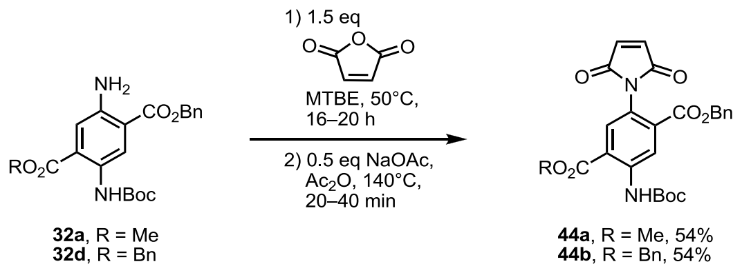
Abbildung 54: Darstellung von NiWa Blue 44a und NiWa Blue 44b .
