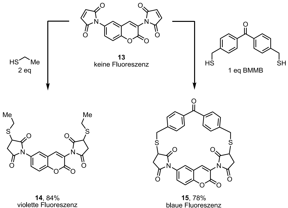
Abbildung 7: Addition von Mercaptoethan und BMMB an das Coumarin-Derivat 13 .
