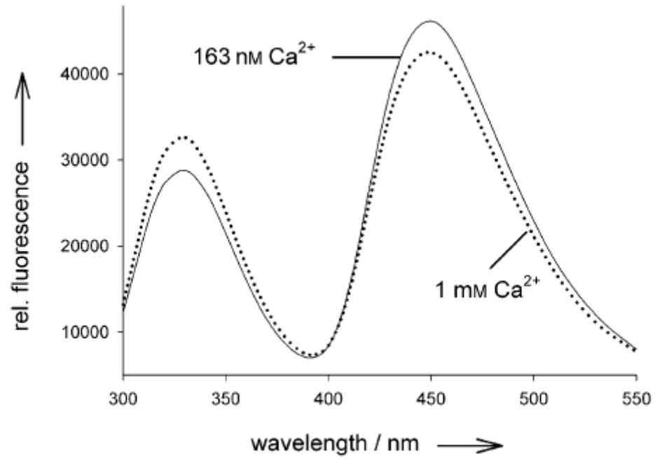
Abbildung 63: FRET-Studie beim markierten Recoverin, \lambda_{irr} = 280 nm.
