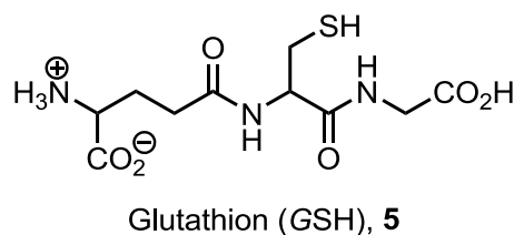
Abbildung 2: Das Pseudotripeptid Glutathion.
