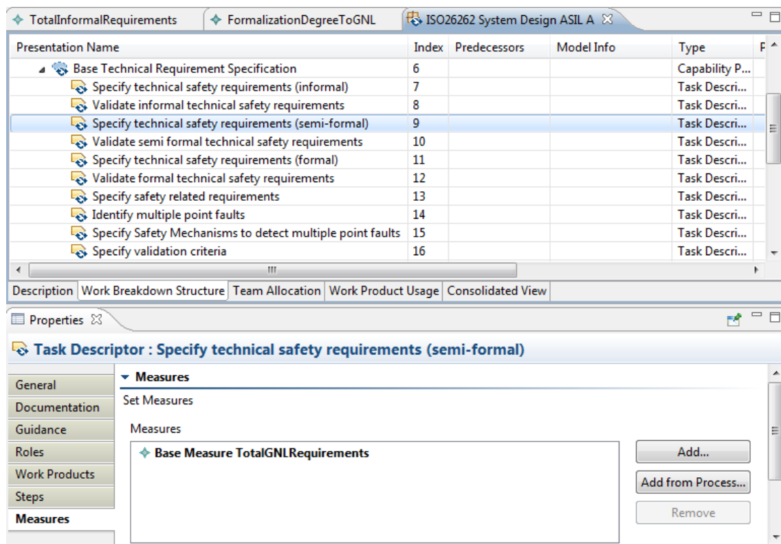
Abbildung 47: Prozessdefinition
