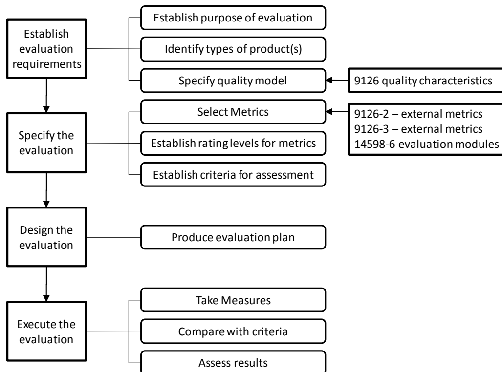
Abbildung 20: ISO 14598 Evaluierungsprozess
