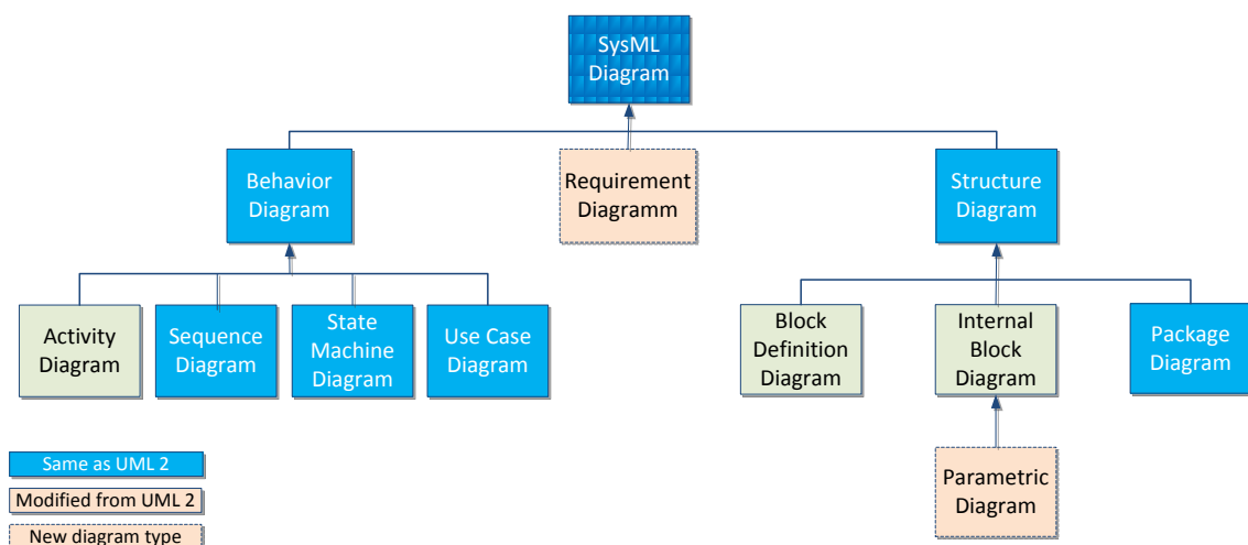
Abbildung 6: SysML Diagramme
